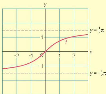
figuur K.9 De functie f(x) = \arctan(x) heeft D_f = \mathbb{R} en B_f = \langle -\frac{1}{2}\pi, \frac{1}{2}\pi \rangle .
