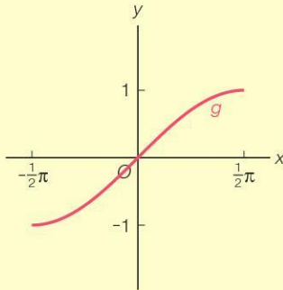
figuur K.13 g(x) = \sin(x) met domein [-\frac{1}{2}\pi, \frac{1}{2}\pi] .
