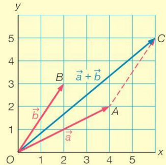
figuur 10.6 De kop-staartconstructie.
