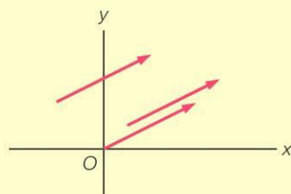
figuur 10.4 Gelijke vectoren.
