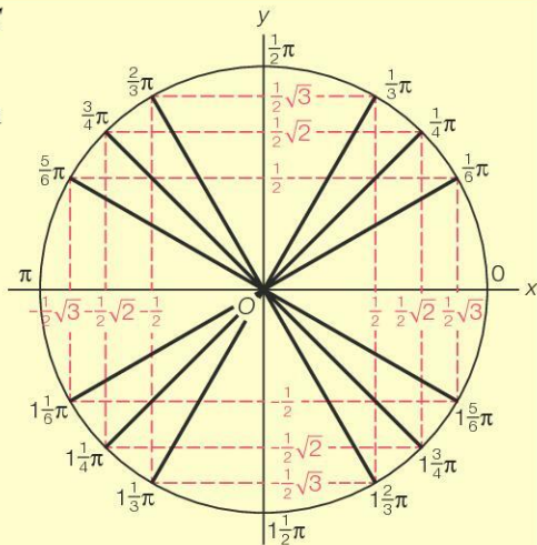
figuur 12.2 De exacte-waarden-cirkel.
