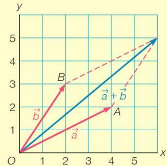
figuur 10.5 De parallellogramconstructie.
