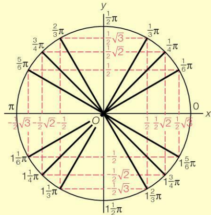
figuur 16.128 De exacte-waarden-cirkel.
