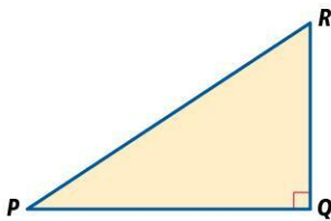
\angle Q = 90^\circ rechthoekige driehoek
